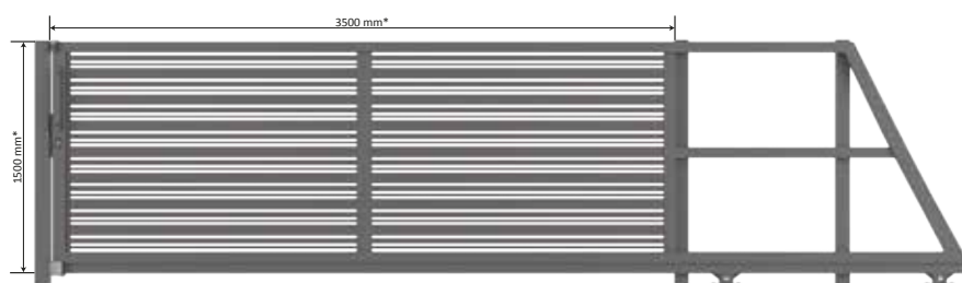
Samonosná posuvná brána DALLS
